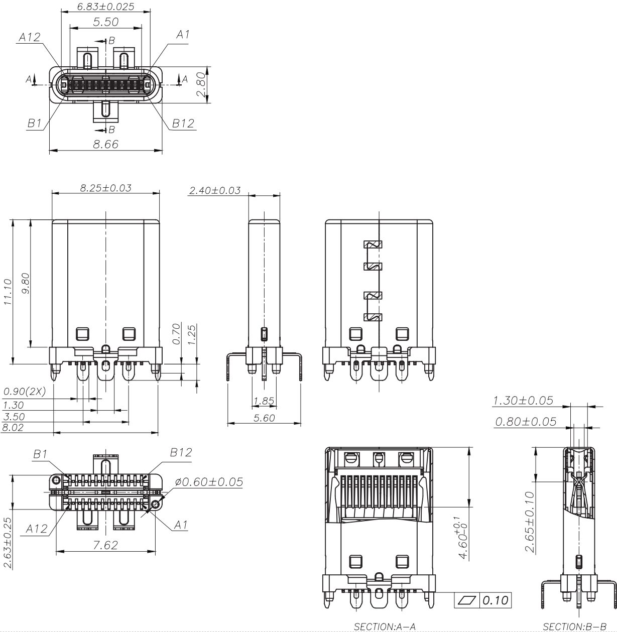
SECTION:A-A
